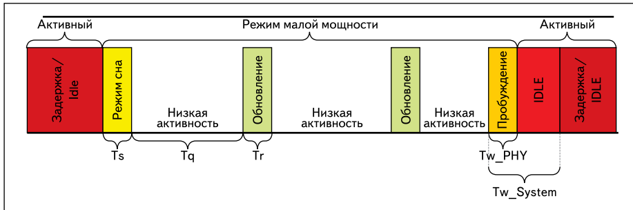
Рис. 7. Пример энергосберегающей работы в Ethernet по IEEE 802.3az
