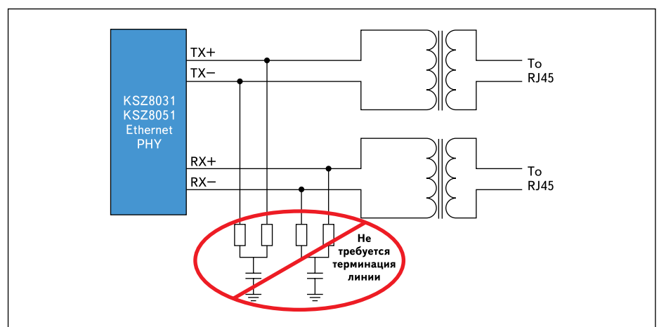
Рис. 2. В микросхемах PHY KSZ8021/31/51 терминирование линии встроено, поэтому нет необходимости в применении дополнительных внешних компонентов
