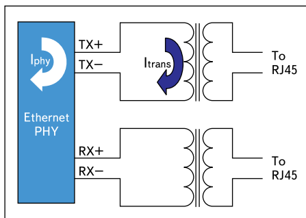
Рис. 1. Рассеяние мощности в цепи Ethernet PHY для режима Current-Mode
