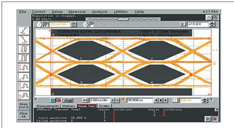
Рис. 6. Глазковая диаграмма сигнала для 100Base-Tx IEEE802.3
