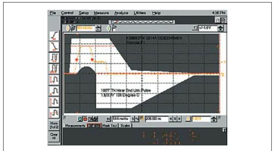
Рис. 5. Импульсы Link Pulse при 10Base-T
