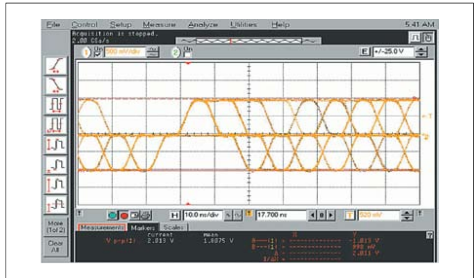
Рис. 4. Паттерн сигнала для 100Base-Tx в состоянии Idle
